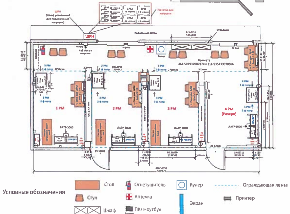
План помещения ИСУЭ для проведения чемпионата WorldSkills на площадке ПАО «Россети Московский регион» по компетенции «ИСУЭ»
